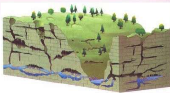
Рис. 160. Карст
