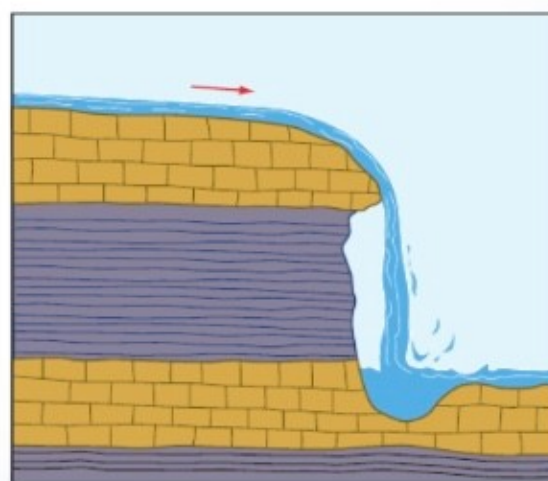
Рис. 81. Схема водопада
