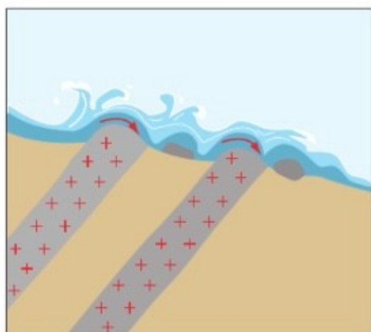
Рис. 80. Схема порогов
