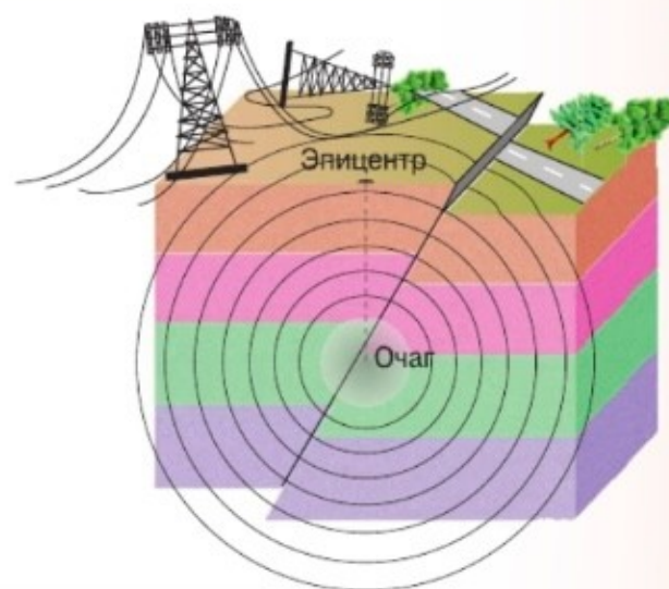
Рис. 57. Схема землетрясения
