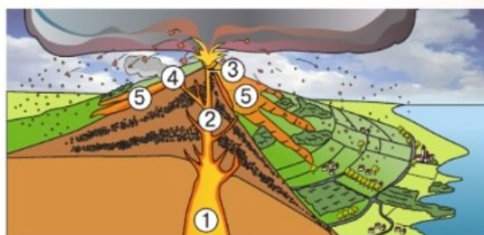
Рис. 59. Строение вулкана: 1 — очаг магмы; 2 — жерло; 3 — кратер; 4 — боковой кратер; 5 — лавовый поток
