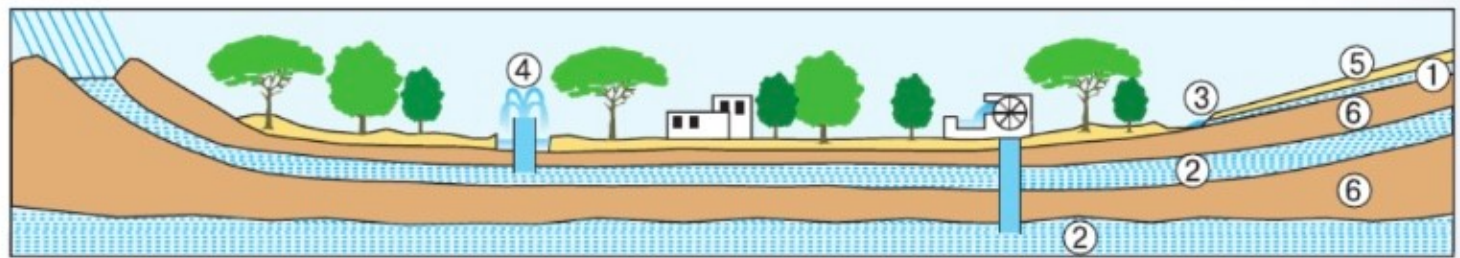
Рис. 85. Подземные воды: 1 — грунтовые воды; 2 — межпластовые воды; 3 — родник; 4 — артезианский источник; 5 — водопроницаемые породы; 6 — водоупорные породы
