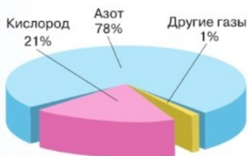
Рис. 89. Состав воздуха
