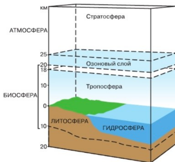
Рис. 109. Границы биосферы
